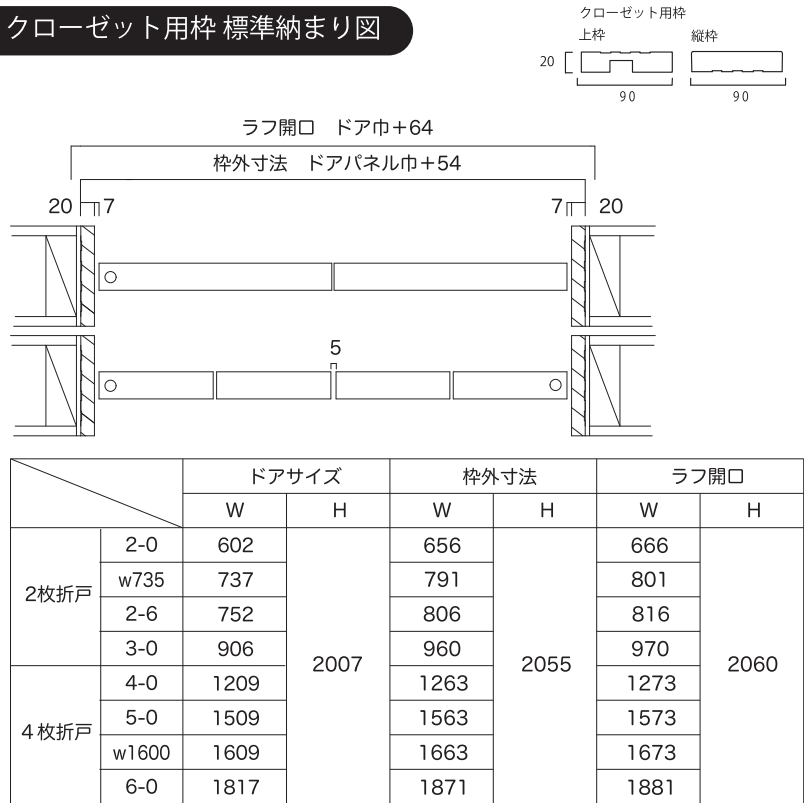
クローゼット用枠 標準納まり図（無目枠）
