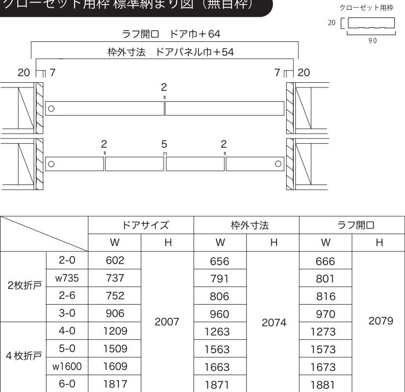
クローゼット用枠 標準納まり図（無目枠）
